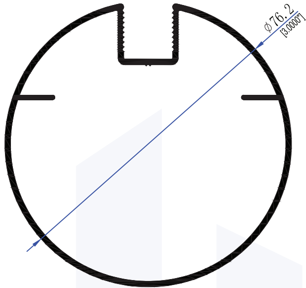
53883 PASAMANOS DE 3"
