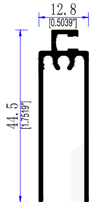
6533 CABEZAL Y ZOCLO MOSQUITERO
